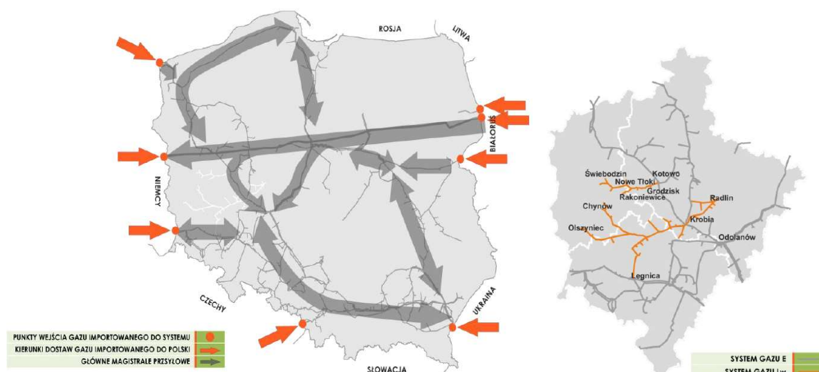
Rysunek 44. Główny układ magistralny gazu E (po lewej) oraz gazu Lw (po prawej), Źródło: Krajowy dziesięcioletni plan rozwoju systemu przesyłowego na lata 2016-2025, GAZ-SYSTEM S.A.
