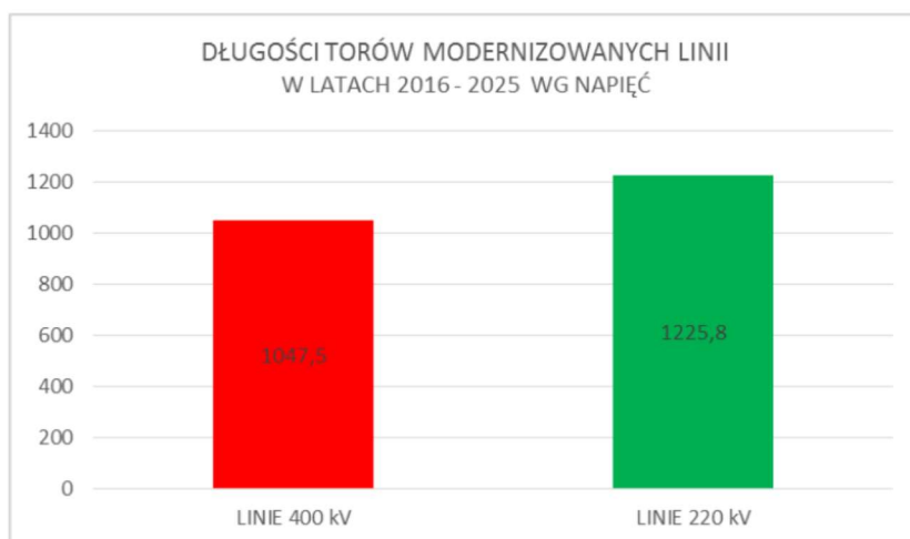
Rysunek 41. Budowa nowych linii przesyłowych NN i likwidacje linii 220 kV na tle linii istniejących [km], Źródło: PSE S.A.
